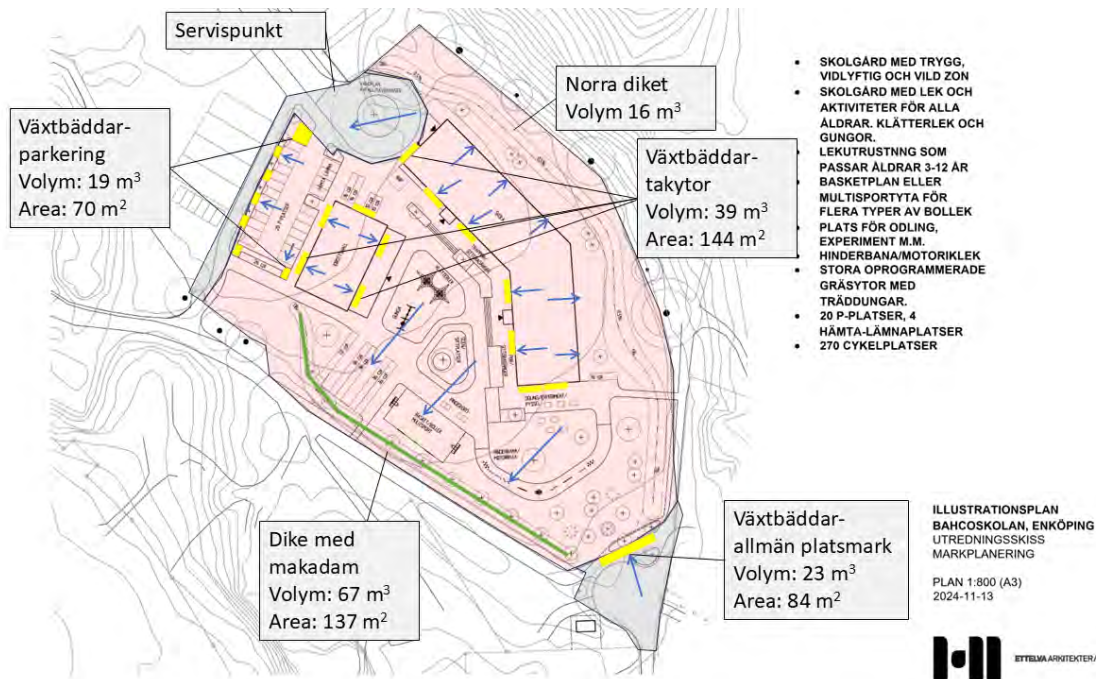
Figur 26. Avvattningsplan för skolområdet. (*Utritade lösningar för delar av allmän platsmark saknas, motsvarande 75 m 2 ). Gråa ytor visar allmän platsmark, rosa ytor är kvartersmark.
