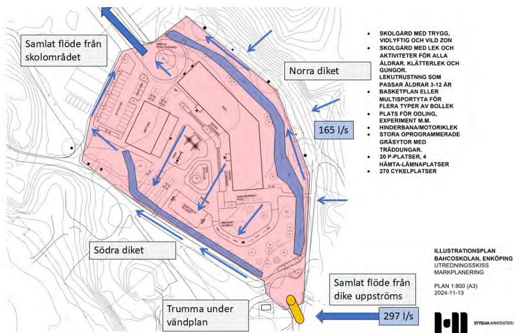
Figur 22. Skyfallsvägar till, inom och från utredningsområdet utifrån planerad exploatering.
