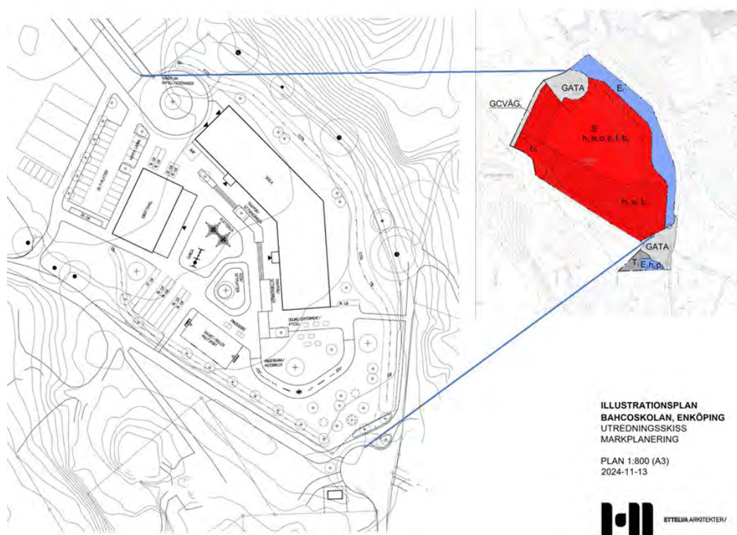
Figur 14. Illustrationsplan erhållen från ETTIELVA ARKITEKTER (2024-11-13). Till höger syns allmän platsmark, markerat med grått och kvartersmark, markerat med rött, det blå markerar skyfallsdike i den norra delen av kvartersmarken.
