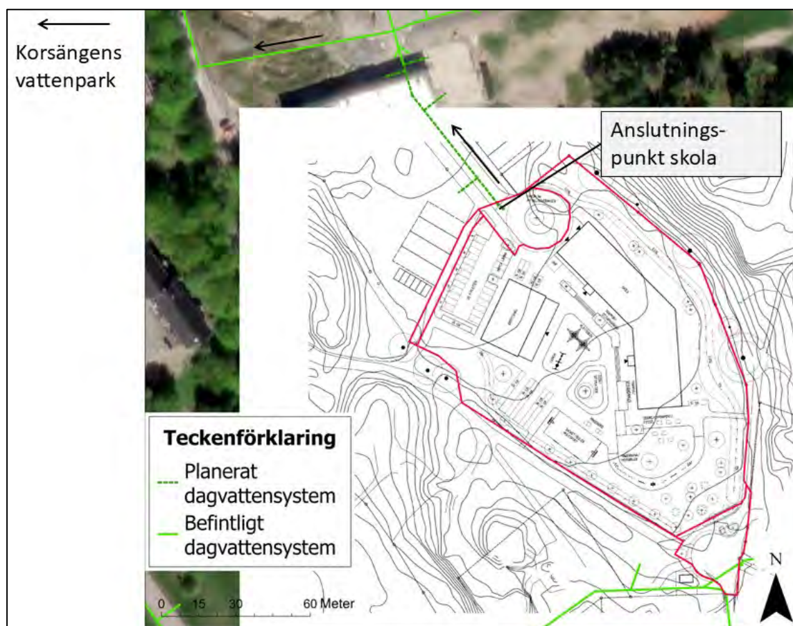
Figur 15. Befintligt ledningssystem i närområdet (gröna heldragna linjer) samt planerad utbyggnad av det kommunala dagvattennätet mot skolan (gröna streckade linjer). Figuren visar även den servispunkt som dagvattnet från skolan planeras att anslutas till. Svarta pilar visar den riktning som dagvattnet har i ledningssystemet.
