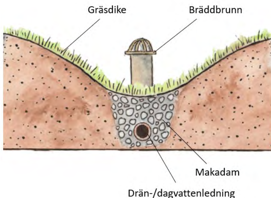
Figur 21. Modifierad bild från original: VA-guiden ( https://vaguiden.se/dagvatten/anlaggningswiki/svackdike/ )
