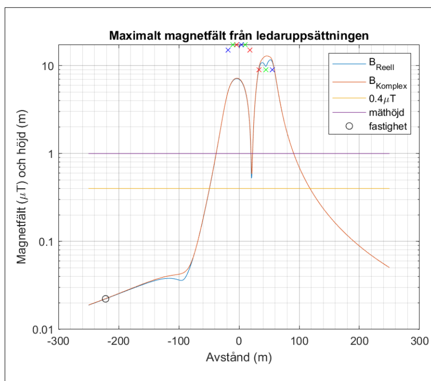
Figur 11: Grafen redovisar den förväntade genomsnittliga magnetfältstyrkan vid normal drift. Kryssen visar vardera faslinan, där röd, grön och blå, avser fas 1, 2 och 3. Beräkningen har genomförts av Svenska kraftnät.
